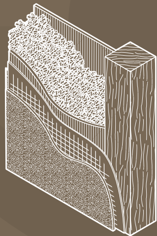
STRUTTURA PARETE
